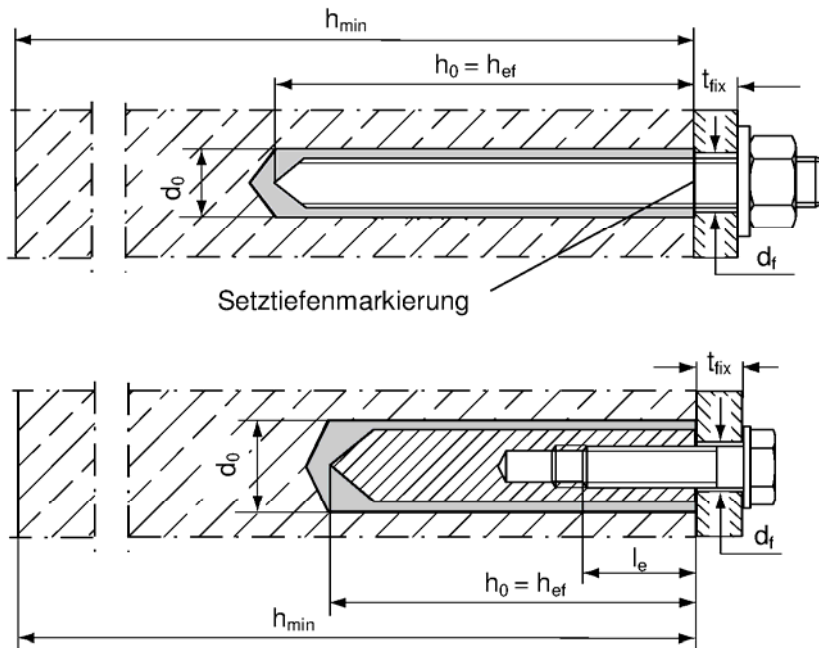
fischer Ankerstange RGM Nur Vorsteckmontage
