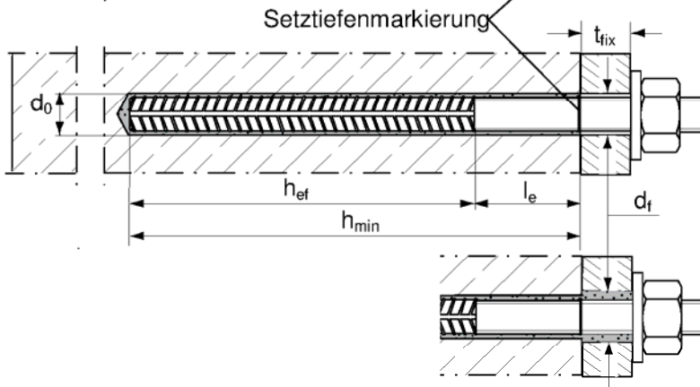
fisher Bewehrungs- Anker FRA
