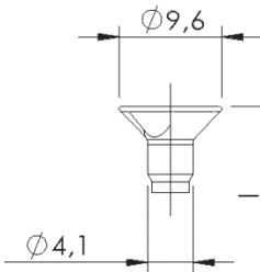
Flachsenkopf mit Kopfloch- bohrung, mit und ohne Frästaschen
