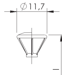
Flachsenkopf 60^\circ / 75^\circ mit und ohne Linse, mit und ohne Fräsrippen
