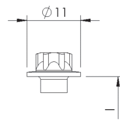
Außensechskantkopf mit und ohne Scheibe
