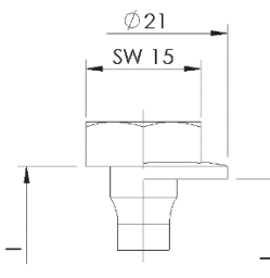
Sechskantkopf mit und ohne Scheibe
