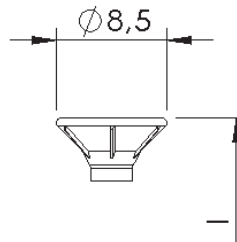
Flachsenkopf mit und ohne Fräsrippen
