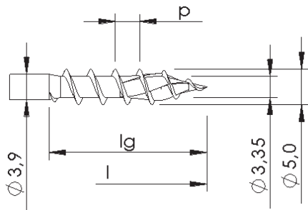
Mit und ohne Gewindevariation, mit Spitzenrippen
