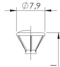
Flachsenkopf 60^\circ / 75^\circ mit und ohne Linse, mit und ohne Fräsrippen
