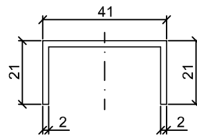
Ansicht C-Profil M 1:1
