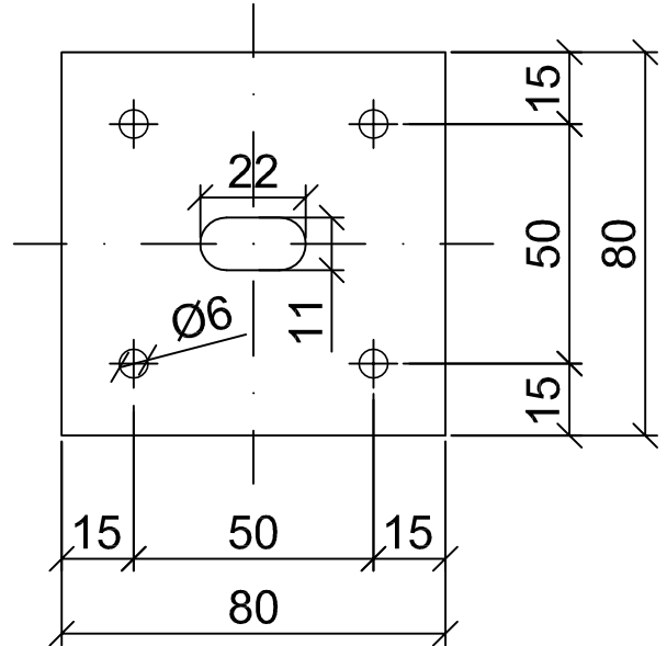
Ansicht obere Platte
