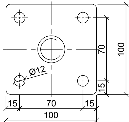
Ansicht obere Platte mit Gewinde M30 links
