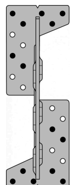
Clouage sur poteau
