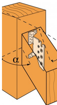
Anschluss mit Neigung und Schräge an Stütze
