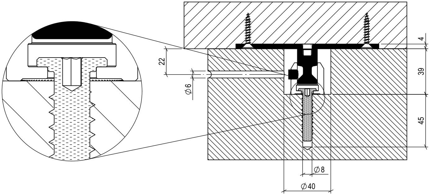
Ansicht A:A
