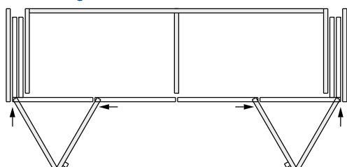
Hawa Folding Concepta III 25 Pull links/rechts Aluminium, eloxiert
