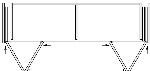
Hawa Folding Concepta III 20 Pull, links/rechts Aluminium, eloxiert
