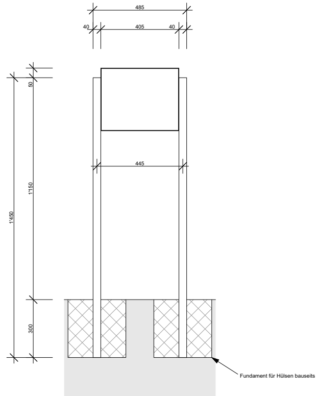
FRONTANSICHT
