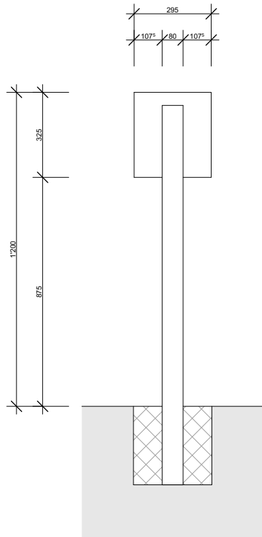
SEITENANSICHT
