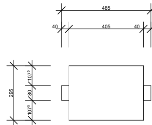
AUFSICHT
