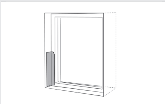
Verkleben des Produktes auf dem Fensterrahmen
