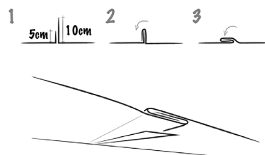
Sigillatura sormonti a soffitto
