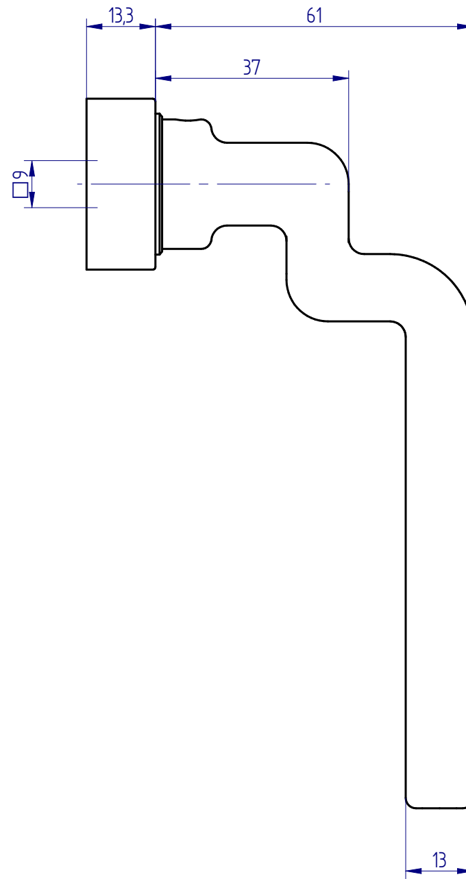
Katalogzeichnung 34190+33605
