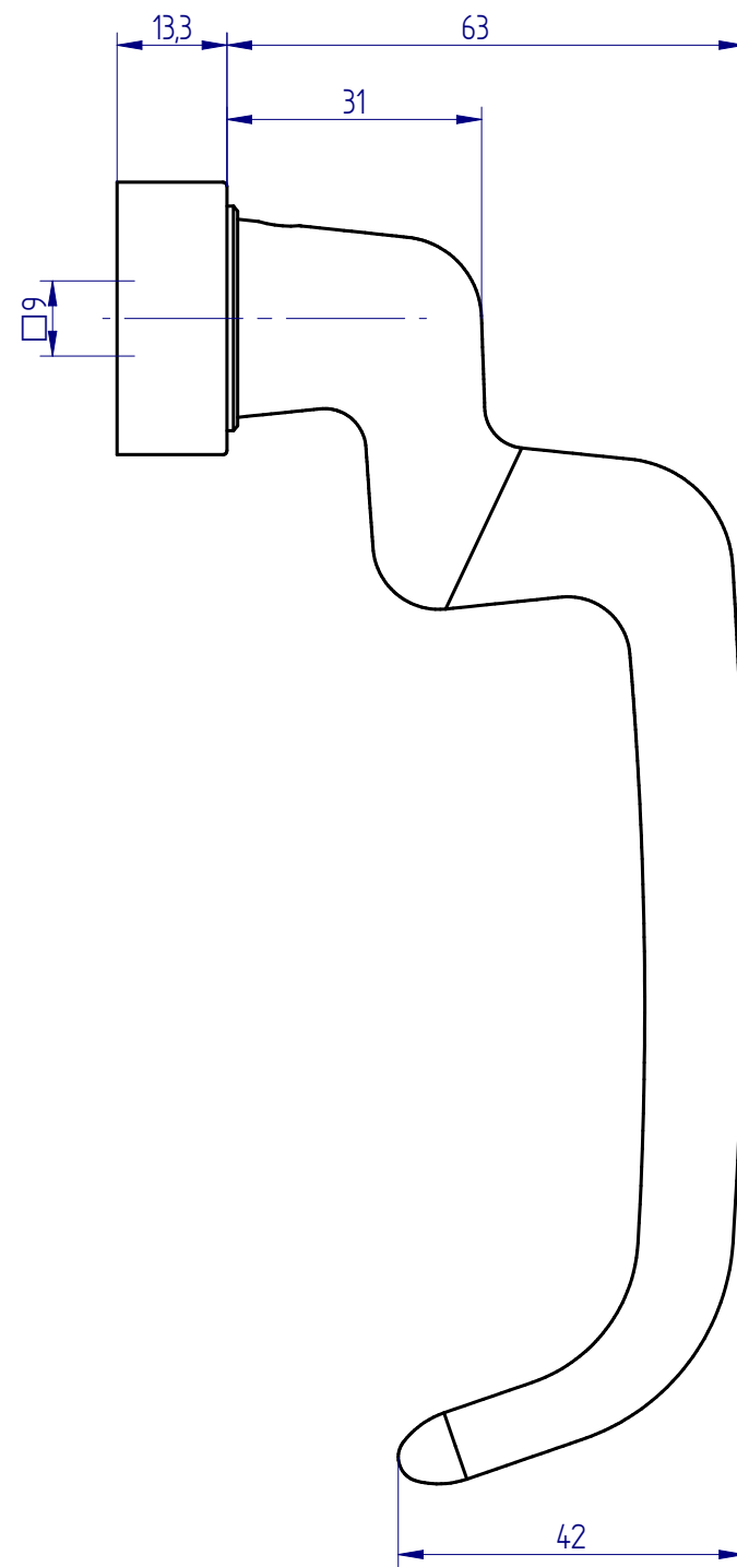
Katalogzeichnung 34190+33104
