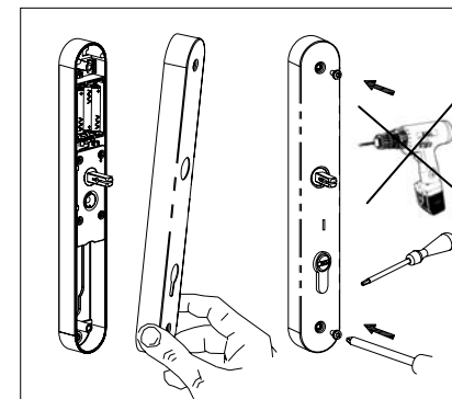
Auswechseln des Spindelsets / Spindle set replacement / Remplacement de la broche / Cambio set mandrino
