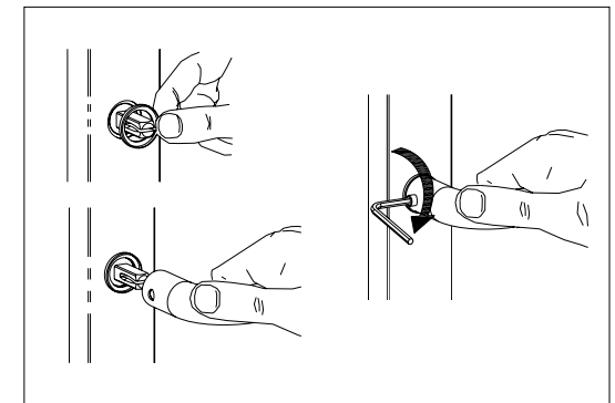
Auswechseln des Spindelsets / Spindle set replacement / Remplacement de la broche / Cambio set mandrino
