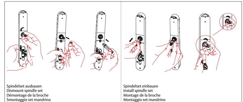
Auswechseln des Spindelsets / Spindle set replacement / Remplacement de la broche / Cambio set mandrino
