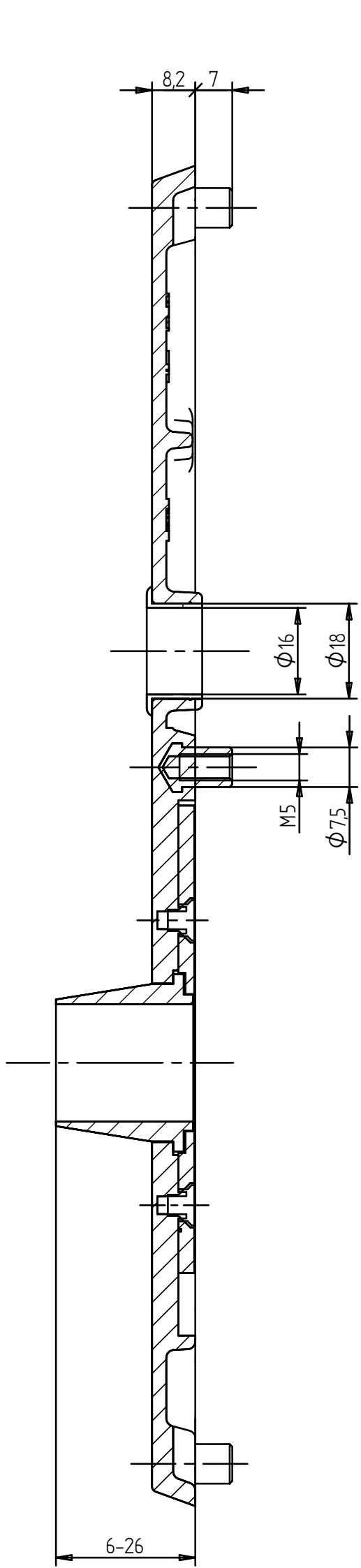
SCHNITT A-A
