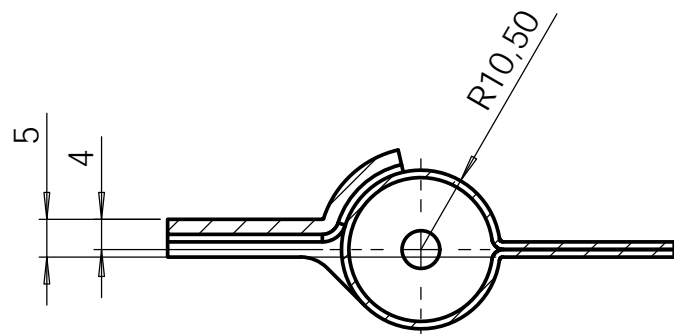
SCHNITT A-A
