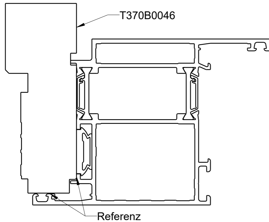
1:2 einwärts öffnende Tür Flügel
