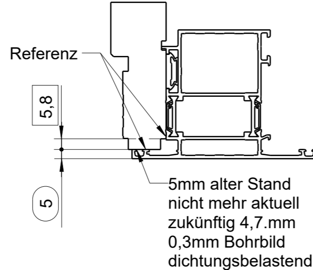
1:2 auswärts öffnende Tür Flügel
