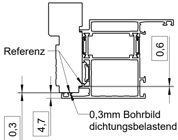
1:2 einwärts öffnende Tür Flügel
