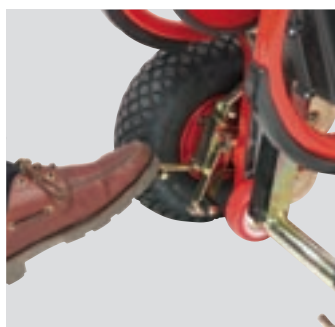
7 Art.-Nr. E/1543.100533 Automatische Bremse
