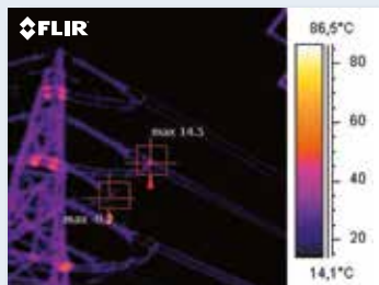
Image de 120 × 120 pixels, sensibilité thermique < 100 mK.
