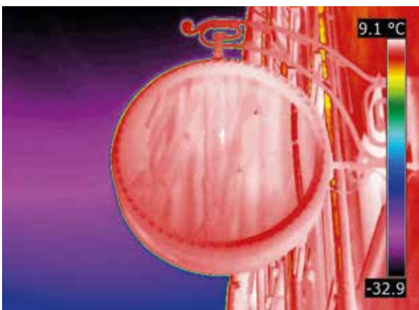
Image thermique sans le mode MSX
